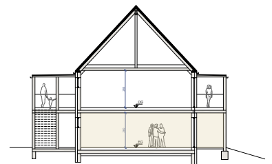
SCHNITT
